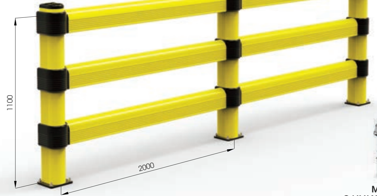
LINK 150/3
